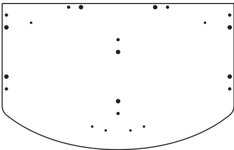
④ Top (DF-00018250) (60 x 38cm)
